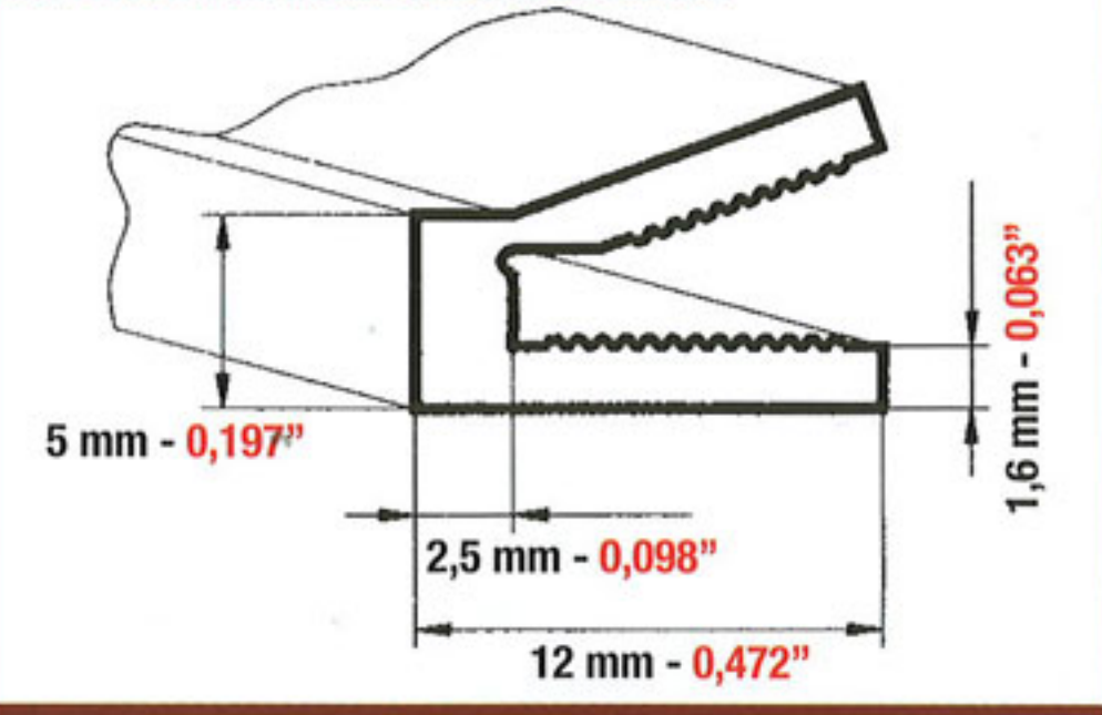
BARRA IN ALLUMINIO ALUMINIUM BAR BARRA EN ALUMINIO 18485
