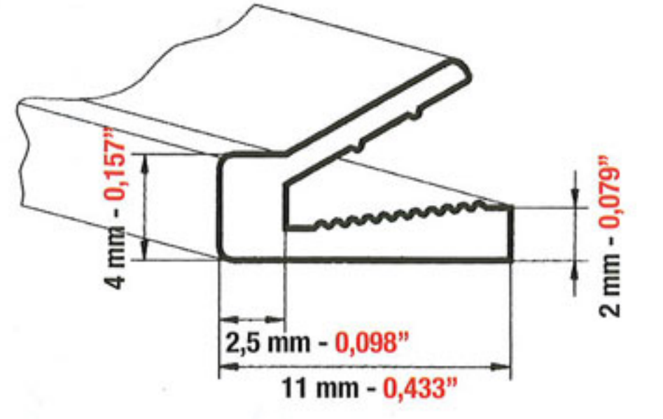
BARRA IN ALLUMINIO ALUMINIUM BAR BARRA EN ALUMINIO 3306
