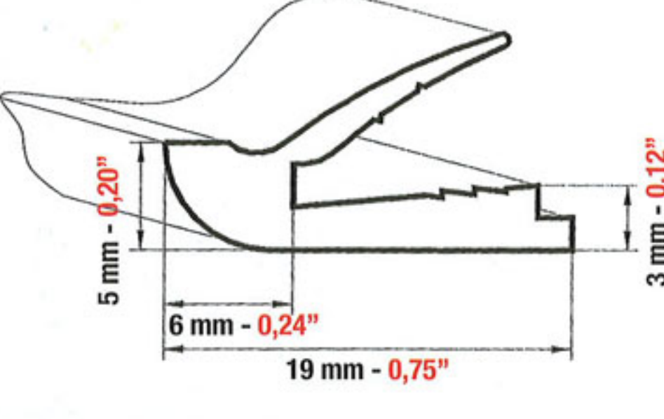
BARRA IN ALLUMINIO ALUMINIUM BAR BARRA EN ALUMINIO 3351
