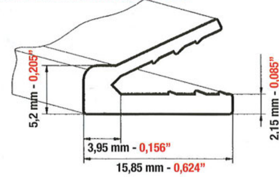
BARRA IN ALLUMINIO ALUMINIUM BAR BARRA EN ALUMINIO 3026
