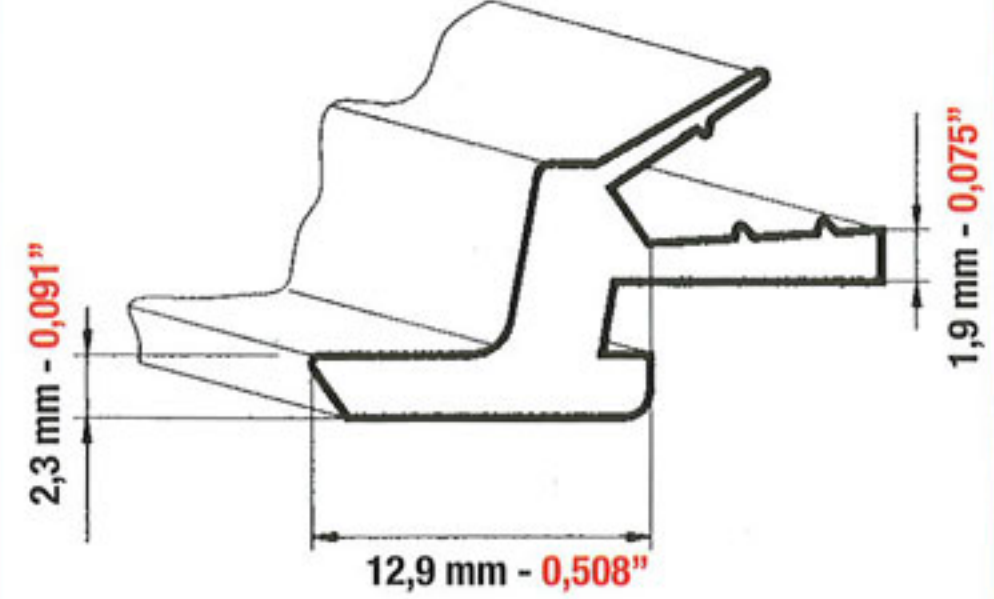
BARRA IN ALLUMINIO ALUMINIUM BAR BARRA EN ALUMINIO 23175 SLAVE BAR
