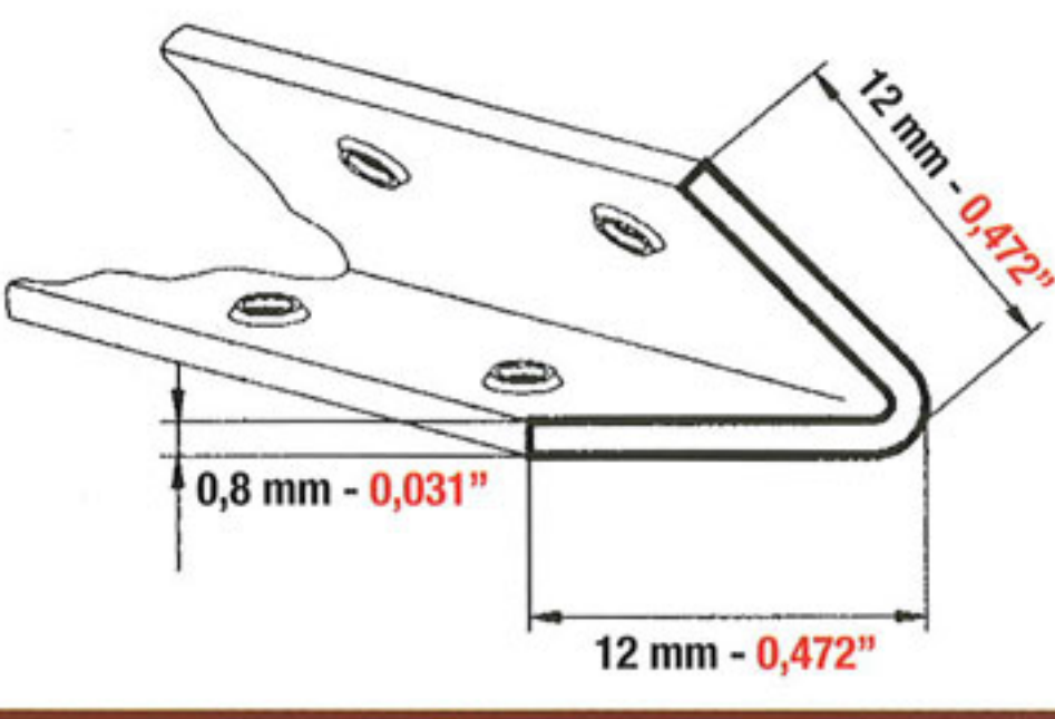
BARRA IN ACCIAIO STEEL BAR BARRA EN ACERO 51208-ZR
