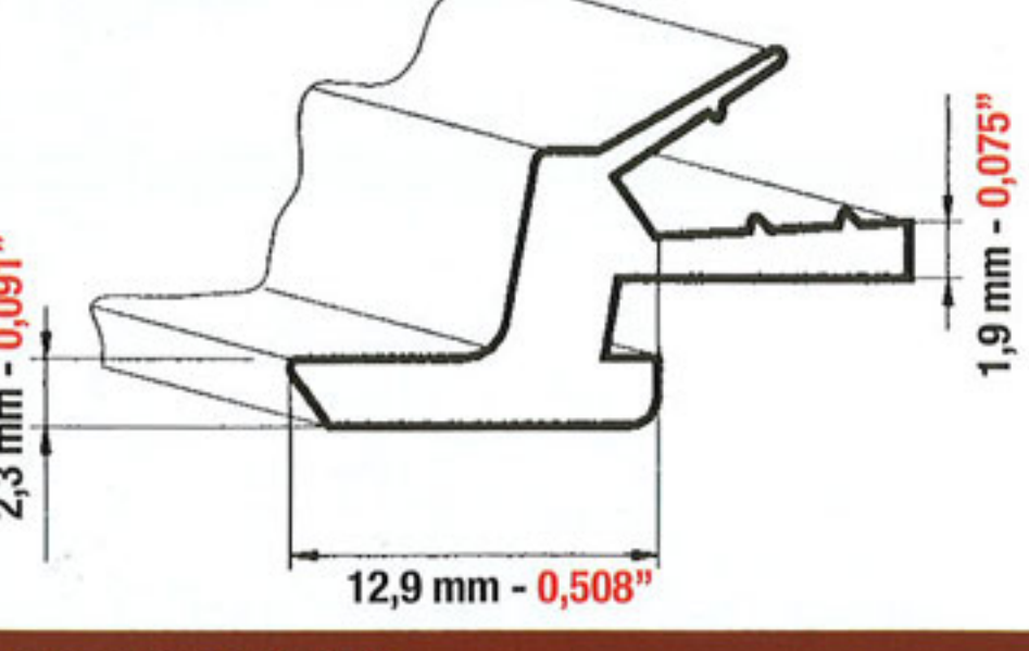
BARRA IN ALLUMINIO ALUMINIUM BAR BARRA EN ALUMINIO 23175
