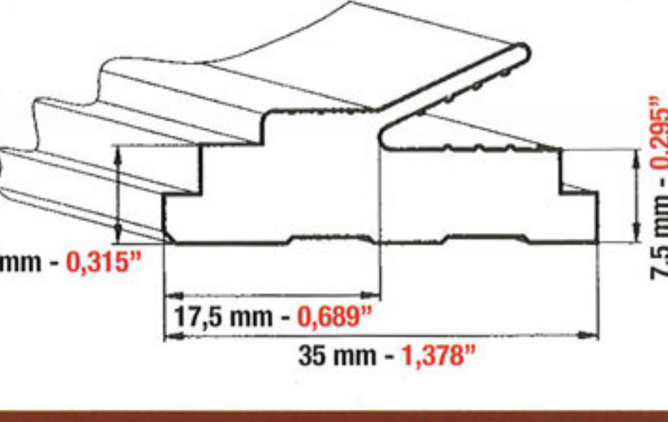
BARRA IN ALLUMINIO ALUMINIUM BAR BARRA EN ALUMINIO 22422
