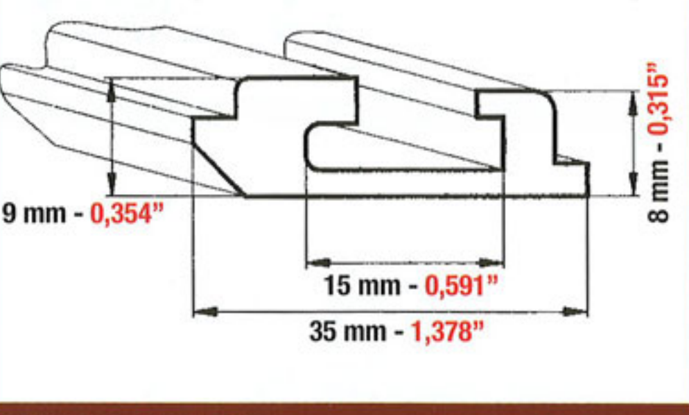
BARRA IN ALLUMINIO ALUMINIUM BAR BARRA EN ALUMINIO MS02
