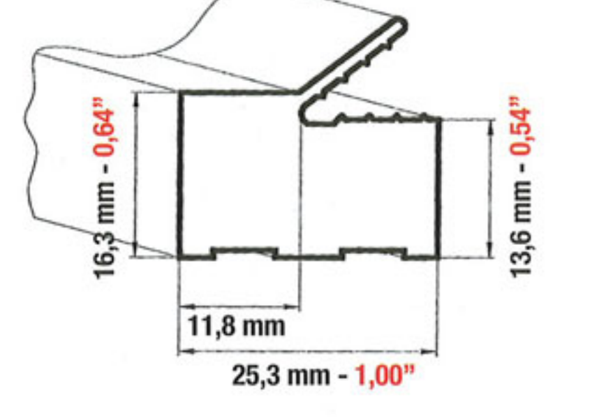
BARRA IN ALLUMINIO ALUMINIUM BAR BARRA EN ALUMINIO 3350
