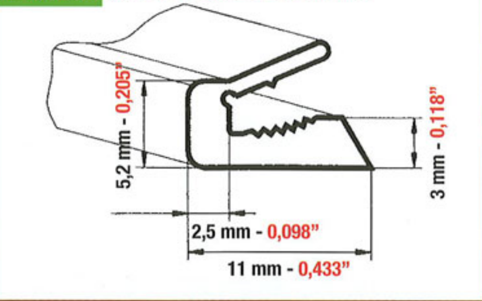
BARRA IN ALLUMINIO ALUMINIUM BAR BARRA EN ALUMINIO 6974
