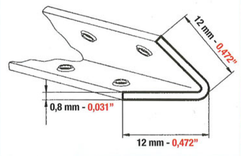
BARRA IN ACCIAIO STEEL BAR BARRA EN ACERO 51208-ZR
