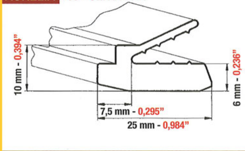
BARRA IN ALLUMINIO ALUMINIUM BAR BARRA EN ALUMINIO 6963
